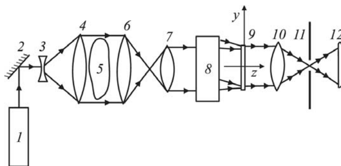
Рис. 1. Оптическая схема голографического интерферометра
