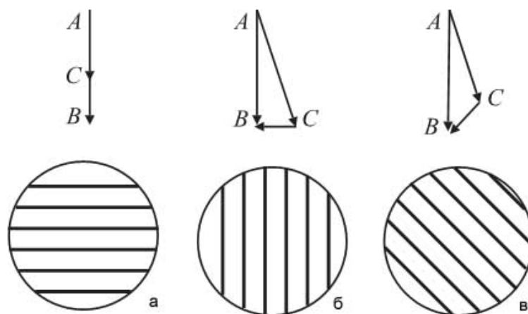
Рис. 2. Векторные диаграммы, поясняющие настройку фоновых полос, и соответствующие им интерференционные картины
