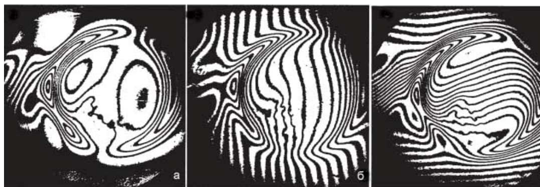
Рис. 3. Интерференционные картины с различной настройкой полос: а – полосы бесконечной и б, в – конечной ширины
