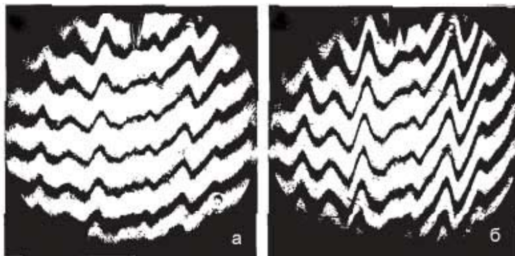
Рис. 4. Интерферограммы, визуализирующие aberrации стеклянных окон камеры, полученные при относительных сдвигах вдоль оси y , равных (а) 0.4 мм и (б) 0.8 мм
