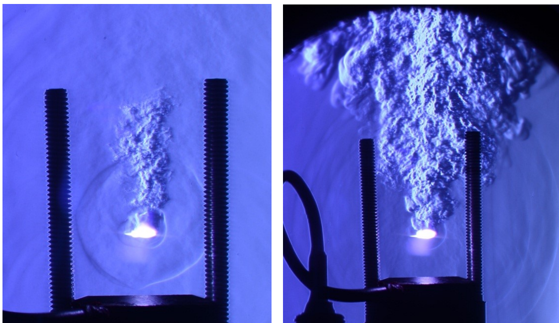
в) г) Рис.6. Иницирование воспламенения метана в дозвуковом потоке
