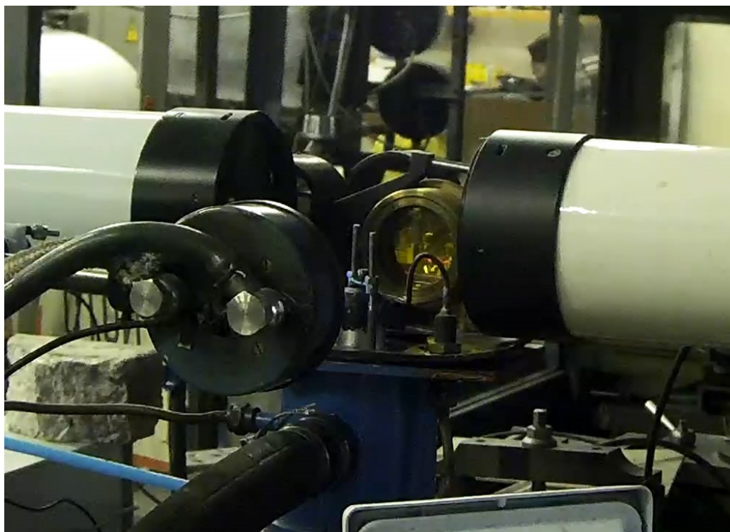
Рис.2. Общий вид эксперимента
