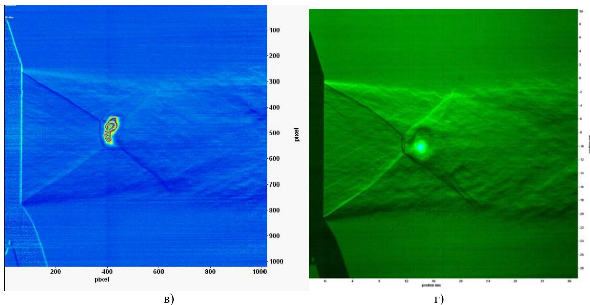
Рис.4. Оптический разряд в сверхзвуковой струе.
