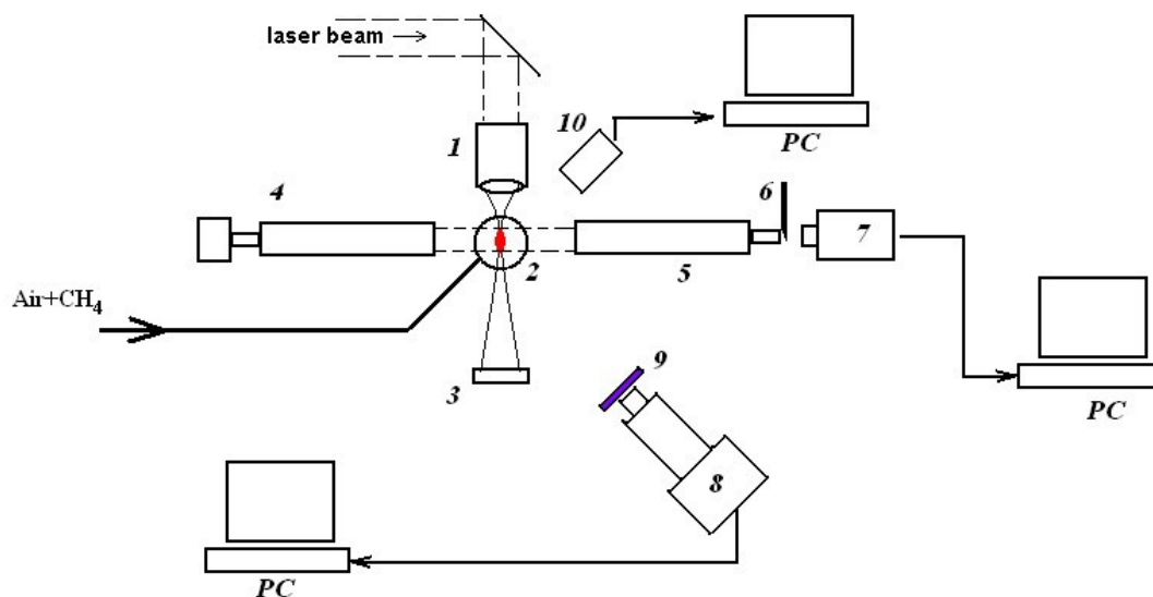
Рис.1. Схема эксперимента: 1 – линзы; 2 – горелка (сверхзвуковое сопло); 3 – поглотитель; 4,5 – шлирен система; 6 – нож; 7 – высокоскоростная камера; 8 – камера спектрозональной съемки; 9 – интерференционный фильтр; 10 – CCD - камера.
